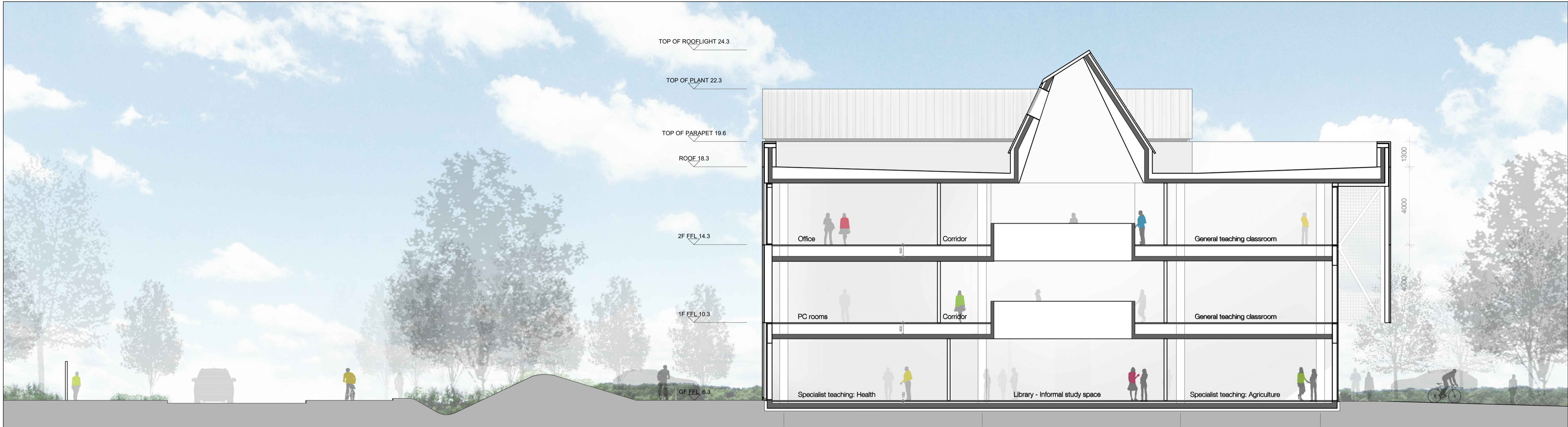
2 Section B 01300 1:100
